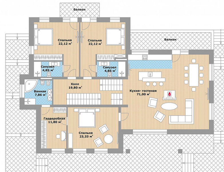
2 ЭТАЖ
