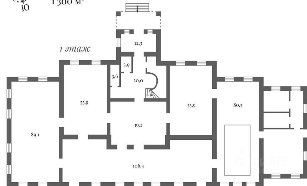
Резиденция в Шульгино 2 этажа и мансарда 1 300 м 2
