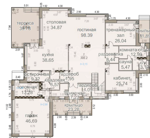
ПЛАН 2 ЭТАЖА
