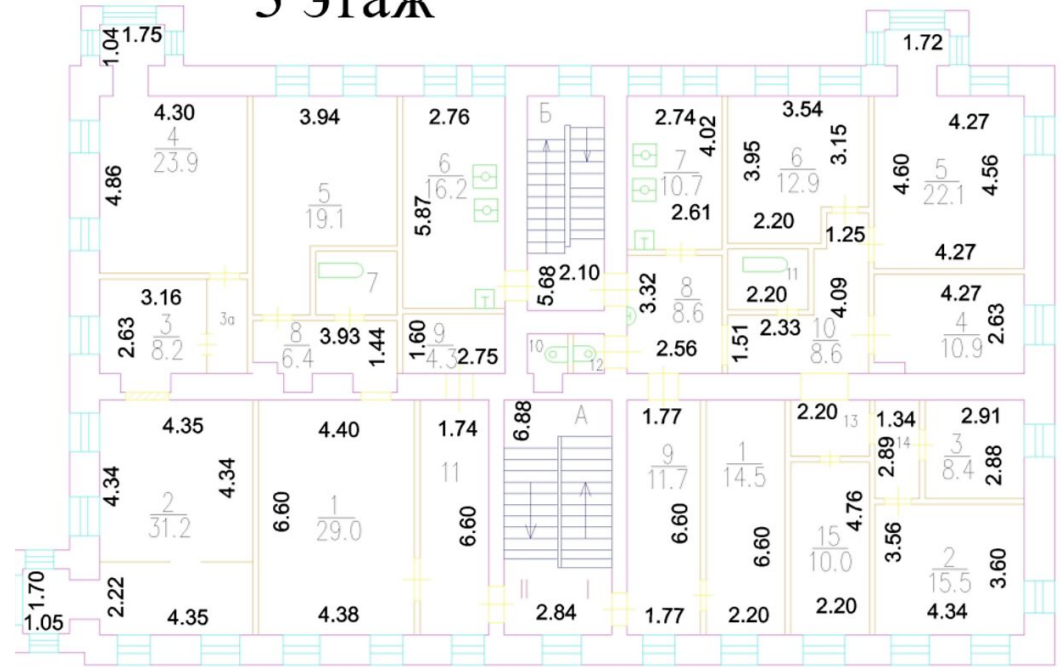
3 этаж
